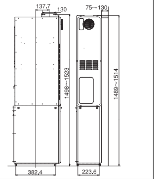
■据置台 ROP-F201 設置図
