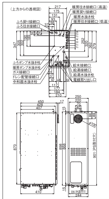
■据置台 ROP-F201 設置図
